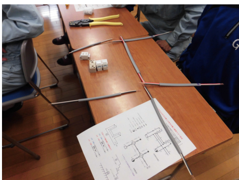
今日の授業材料 (階段のスイッチ)
